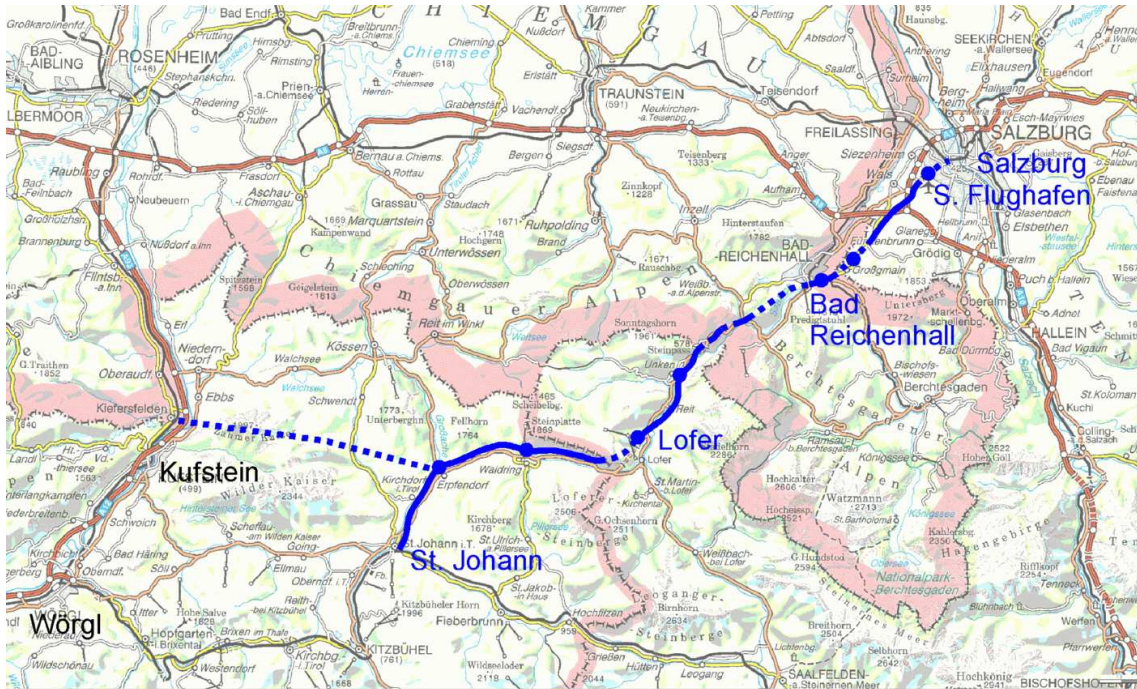
Abb. 10: Eisenbahn-Neubaustrecke St. Johann - Lofer - Salzburg (Konzeption und Grafik: VIEREGG-RÖSSLER GmbH)
