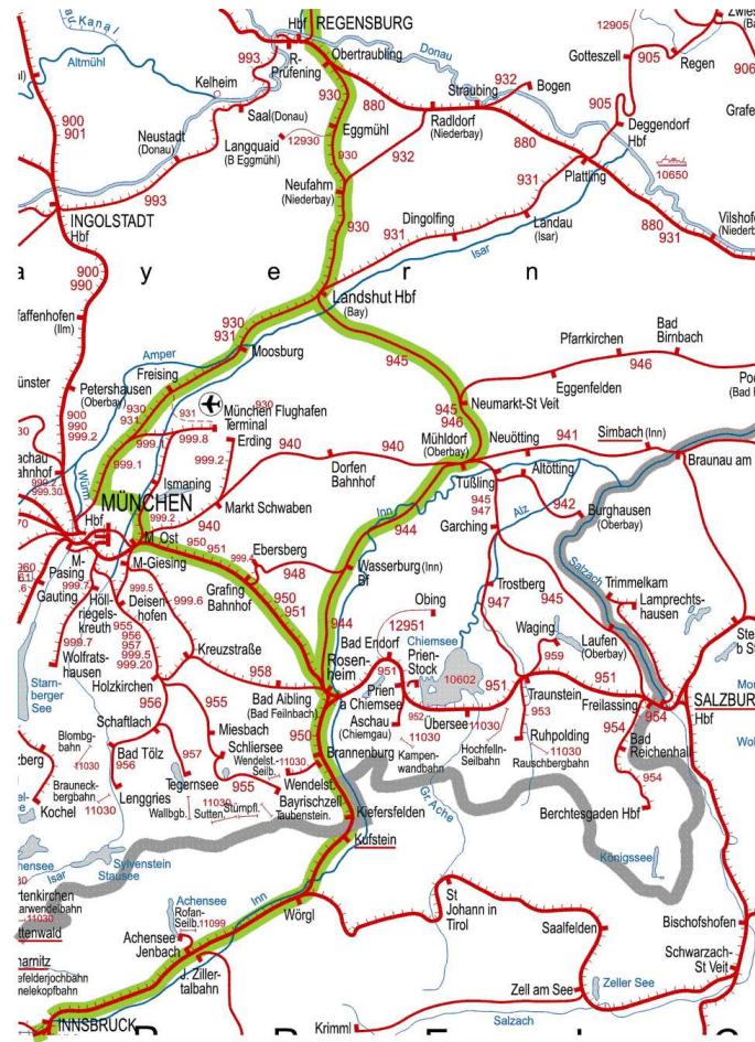
Abb. 4: Mögliche Güterzugleitwege Nord - Süd (Brenner-Zulauf) Regensburg - Rosenheim (Kartengrundlage: DB-Kursbuchkarte)
